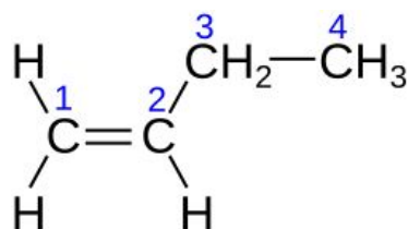
1-butene(C 4 H 8 )
